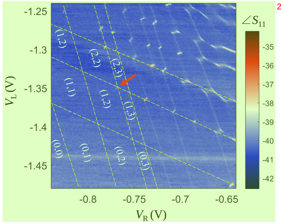
图 4.2 大范围扫描电极电压 V_L 和 V_R ，测量腔相位得到的电荷稳定图。箭头指出了我们实验中的工作区域，在 (1,3)–(2,2) 电荷区。
