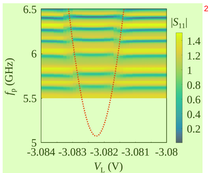
图 3.17 SQUID 阵列谐振腔反射信号 |S_{11}| 在不同腔频下，随探测频率 f_p 和电极电压 V_L 的变化关系。水平方向的深色线对应不同磁通下 SQUID 阵列谐振腔的腔频，在与比特共振交点处会发生腔频偏移。红色虚线为拟合共振点得到的比特跃迁能级。 3
