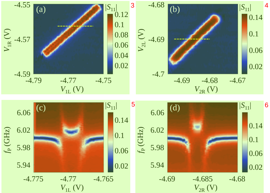
图 3.12 电子隧穿线与真空 Rabi 劈裂。(a)–(b) DQD1 和 DQD2 的量子点间电子隧穿导致的腔幅值信号 |S_{11}| 变化。(c)–(d) 沿图 (a) 与图 (b) 中横向虚线测量的真空 Rabi 劈裂图。
