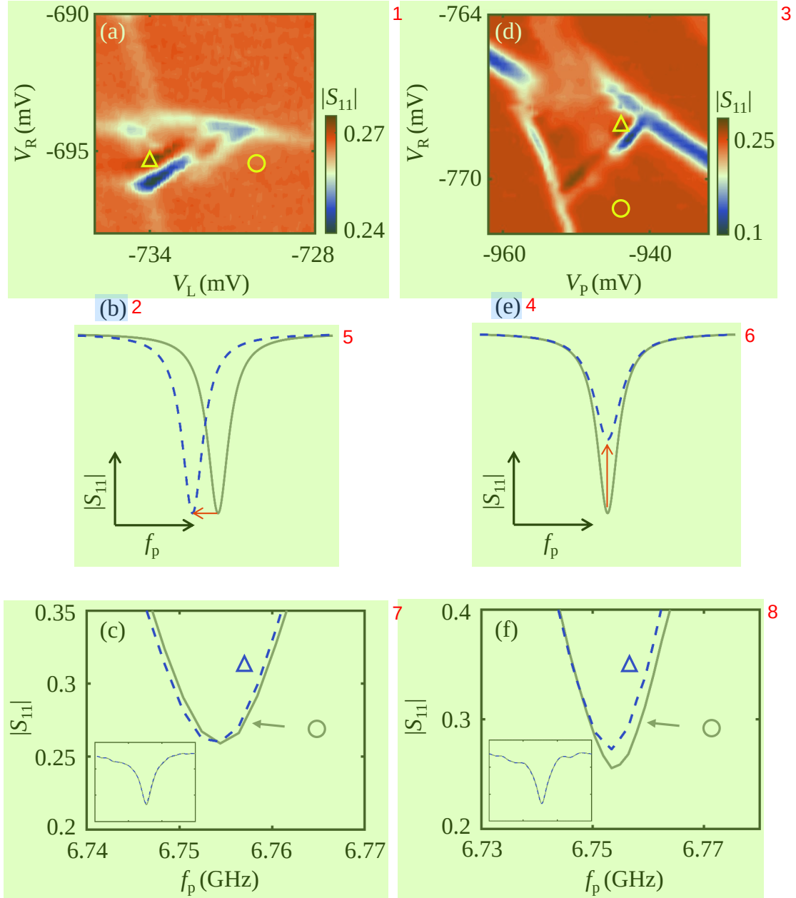
图 5.4 (a),(d) V_{SD} = 0.5 \text{ mV} 时测量腔幅值信号得到的电荷稳定图，用三角形标记出了增益区域，用圆形标记出了库伦阻塞区。(b),(e) 腔频偏移与量子点发光导致的腔信号幅值增益示意图。(c),(f) 在增益区域（虚线）和库伦阻塞区（实线）测量得到的频谱信号，放大展示了谐振谷附近的细节。左下角插图为完整的频谱曲线，几乎重叠在了一起。
