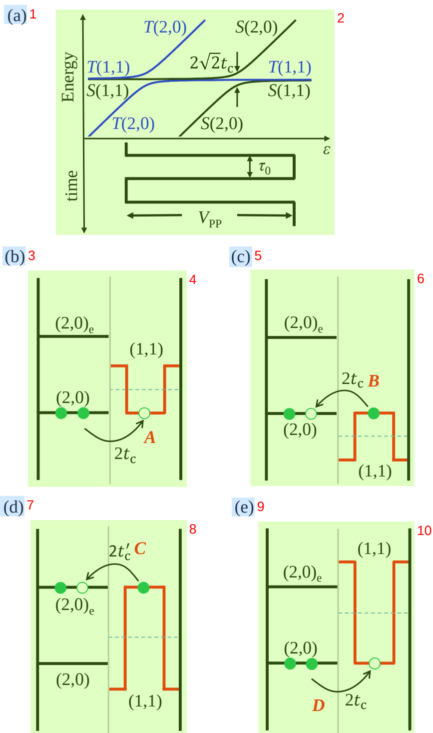
图 4.5 给双量子点施加方波脉冲后，电子的能级跃迁示意图。(a) 上侧：无外加磁场时的双电子自旋态的能级示意图。下侧：方波脉冲引起失谐量 \varepsilon 随时间变化的示意图。(b)–(e) 在图 4.4(a) 中跃迁线 A、B、C 和 D 对应的能级跃迁示意图。
