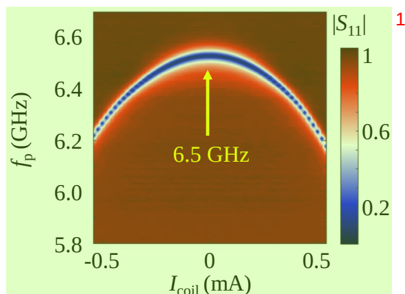
图 3.10 SQUID 阵列谐振腔的谐振频率随线圈电流 I_{\text{coil}} 的变化关系。 2
