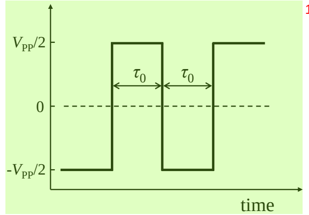
图 4.3 方波脉冲及其参数。 2
