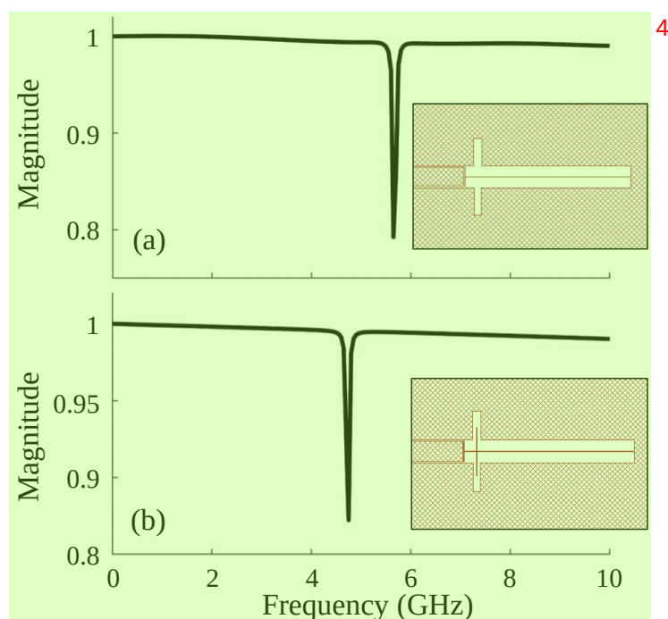
图 3.4 使用“Sonnet”模拟软件模拟耦合电极对腔反射频率谱的影响。(a) 无耦合电极。(b) 有耦合电极。
