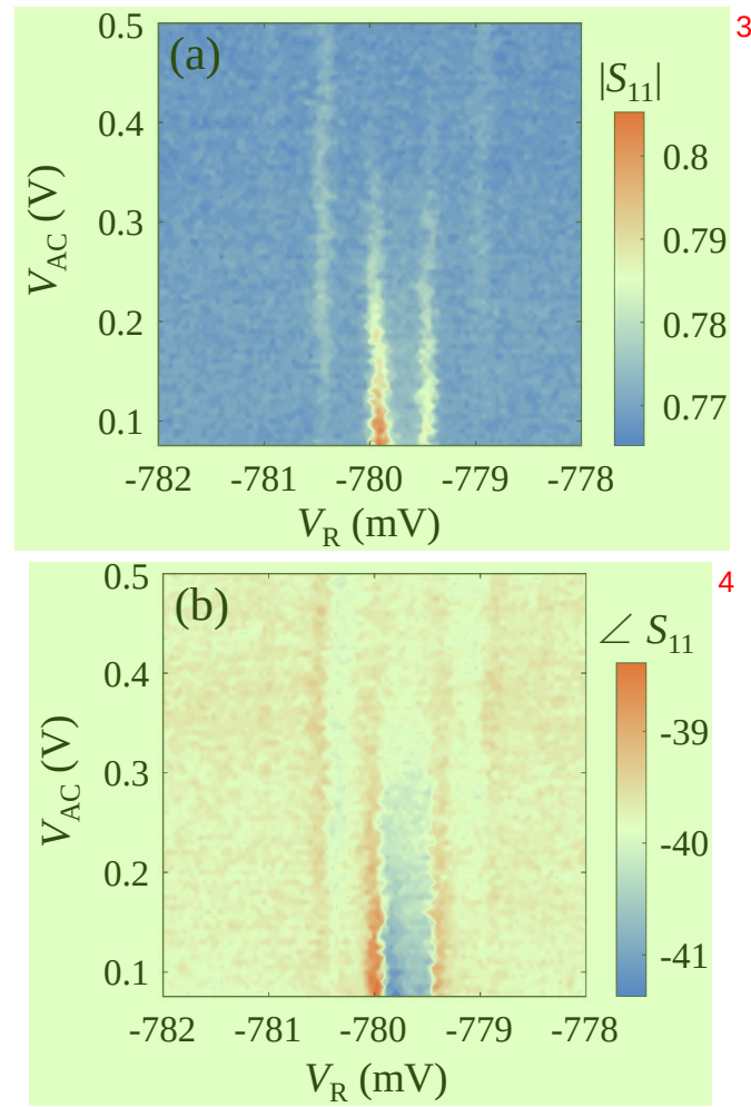
图 3.15 改变量子点电极电压 V_R 与微波幅值 V_{AC} ，利用超导腔探测的双量子光子辅助隧穿谱。(a) 幅值信号谱，(b) 相位信号谱。
