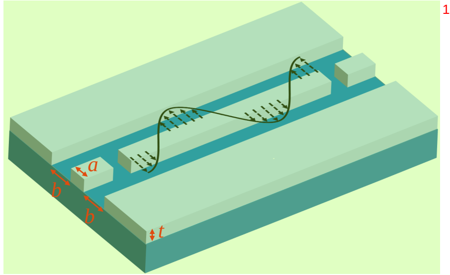
图 2.7 共面波导传输线谐振腔示意图。中心导体线宽为 a ，导体到地平面的距离为 b ，膜厚为 t 。
