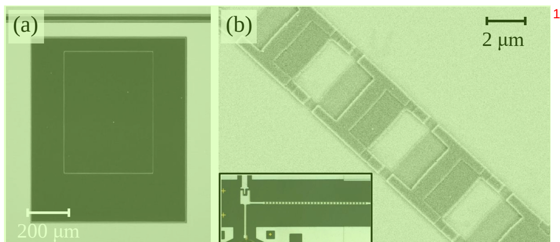
图 1.2 高阻抗超导谐振腔的扫描电子显微镜图。(a) 由 8 nm 厚的 NbTiN 薄膜制备而成的纳米线腔，线宽为 100 nm，围成了矩形形状。白色为 NbTiN 薄膜，黑色对应薄膜被刻蚀掉之后的衬底颜色。图片引自 [61]。(b) 超导量子干涉器件阵列构成的微波腔。左下角插图量子点与腔耦合的整体结构图。图片引自 [51]。
