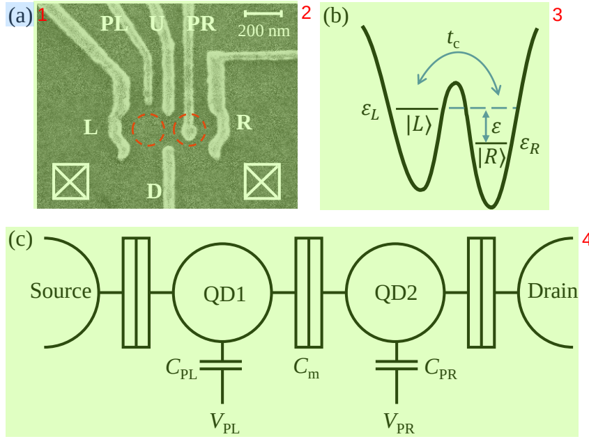
图 2.4 (a) 量子点金属电极电镜图。通过给电极 L、PL、U、PR、R 和 D 施加合适的偏置电压， 会在两个虚线圆圈所指示的位置处形成量子点。(b) 双量子点束缚势示意图。电荷态 |L\rangle 和 |R\rangle 之间以隧穿速率 t_c 耦合，两点之间的电势差为失谐量， \epsilon_L - \epsilon_R = \epsilon 。 (c) 双量子点电路示意图。两点之间通过电容相互耦合，并各自耦合到相邻的源漏 上。通过电极 PL 和 PR 和可以调节两个点内的电势。
