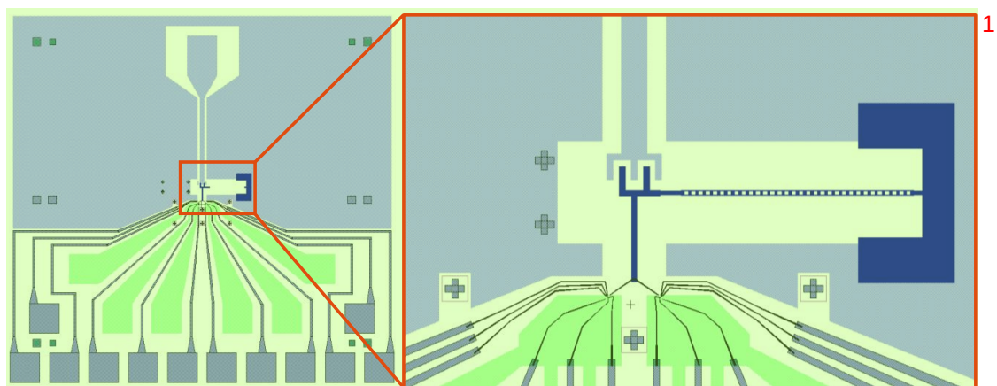
图 3.1 SQUID 阵列谐振腔和 GaAs 两个双量子点耦合结构的设计图。 2
