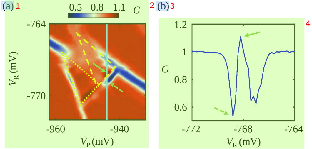
图 5.3 (a) 源漏偏置 V_{SD} = 0.5 \text{ mV} 时，以电极电压 V_P 和 V_R 为扫描参数，测量腔信号增益 G 得到的稳态图。其中上侧的偏压三角形轮廓由虚线标出，下侧的偏压三角形轮廓由点线标出。实线箭头所指的区域腔信号幅值增强， G > 1 ；虚线箭头所指的区域腔信号幅值被抑制， G < 1 。(b) 沿图 (a) 中 V_P = -944 \text{ mV} 截取的一条竖线。尖峰处对应光子发射，而左侧低谷对应光子吸收。
