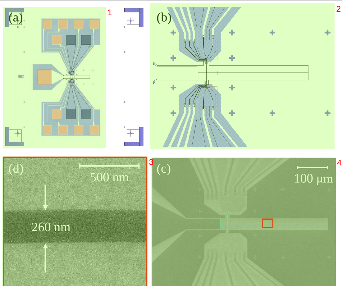
图 3.3 NbTiN 纳米线腔与 GaAs 两个双量子点耦合结构。(a) 结构设计图。(b) 设计图的核心结构放大。(c) 样品的扫描电子显微镜图。(d) 放大后的 NbTiN 腔中心导体，宽度为 260 nm。
