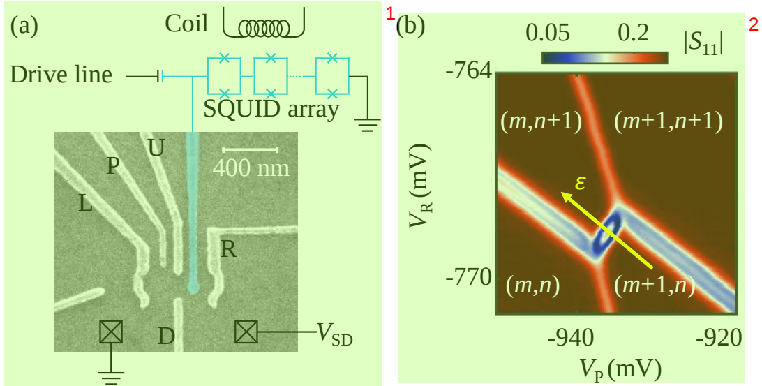
图 5.1 (a) 样品的扫描电子显微镜图。通过给金属电极 L、P、U、R 和 D 施加负偏置电压形成双量子点，同时在源漏上加直流电压 V_{SD} 来驱动双点。量子点的右侧电极连接到 SQUID 阵列构成的谐振腔上，通过测量馈线上谐振腔反射的微波信号可以测得量子点的电荷态。(b) 在 V_{SD} = 0 时，测量 SQUID 腔幅值信号 |S_{11}| 得到的双量子点电荷稳定图，可以观察到双点与源漏之间的隧穿信号，以及量子点之间正斜率的电荷跃迁线。失谐量 \varepsilon 由垂直于量子点间隧穿线的箭头标出。
