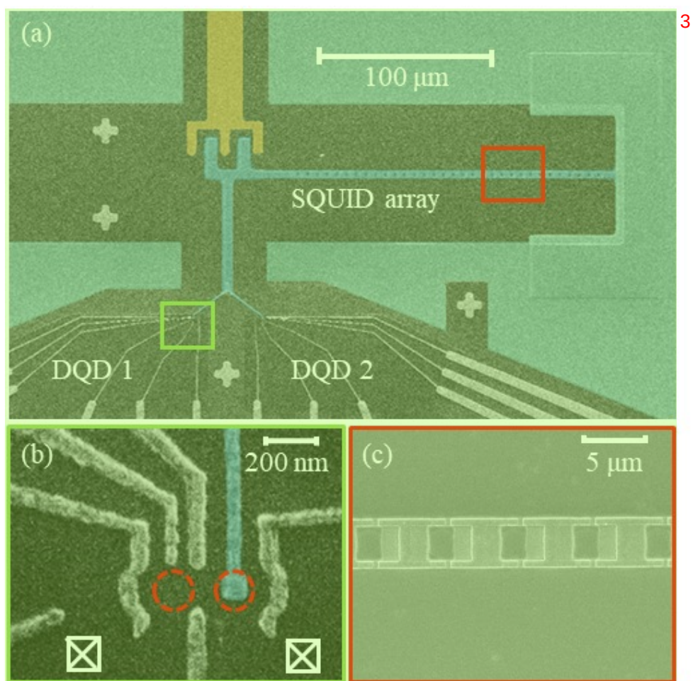
图 3.2 SQUID 阵列谐振腔和 GaAs 两个双量子点耦合样品的扫描电子显微镜图。(b) 和 (c) 分别是图 (a) 中放大的双量子点结构和 SQUID 阵列结构。 4
