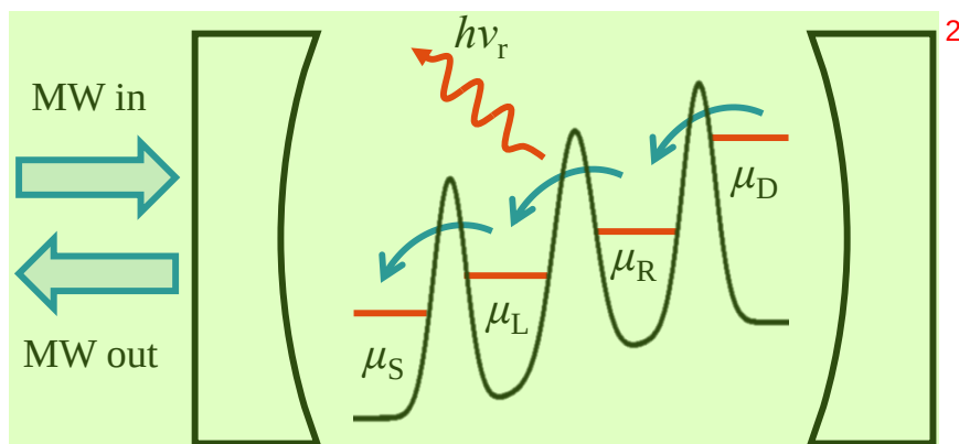
图 5.2 量子点发光模型示意图。双量子点被置于谐振腔内，在源漏驱动下发生电子的连续 2 跃迁发出光子。 3
