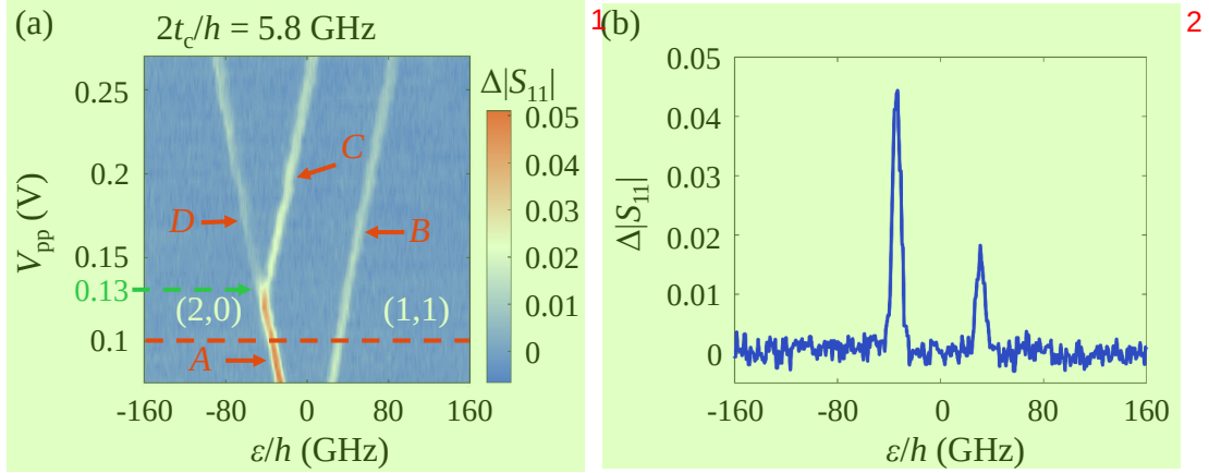
图 4.4 (a) 反射幅值信号 \Delta|S_{11}| 随失谐量 \varepsilon 和脉冲电压 V_{pp} 变化的激发谱，数据已经经过处理扣除了库伦阻塞区的本底。(b) 沿幅值谱图中 V_{pp} = 0.1 \text{ V} 的水平截线。
