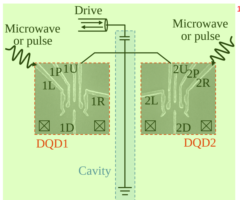
图 3.7 NbTiN 反射腔与两个双量子点耦合的结构示意图。可以给量子点的势垒电极施加微波或脉冲信号。
