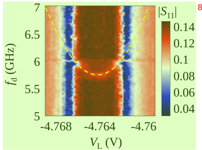
图 3.16 扫描电极电压 V_L 和驱动微波频率 f_d 得到的 two-tone spectroscopy。图中虚线对应量子点能级随电极电压的变化。
