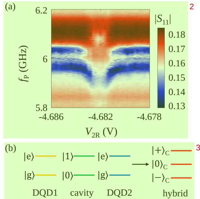
图 3.14 (a) 两比特与腔共振的真空 Rabi 劈裂。(b) 两个双量子点与腔共振时的能级示意图。
