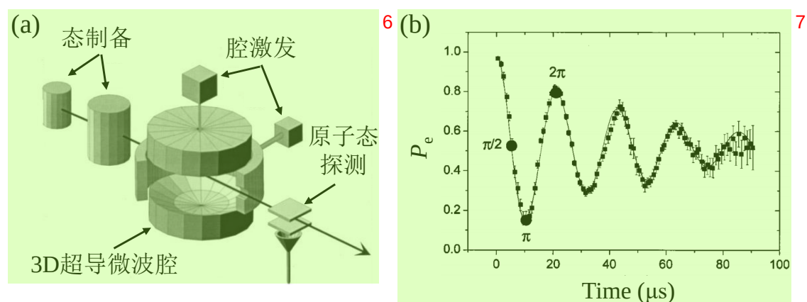
图 1.1 腔量子电动力学的 Rydberg 原子实验。(a) 样品装置图。原子在左侧被初始化到激发态上, 然后经过一个 3D 微波谐振器并被冷却到 \sim 1\text{ K} , 与腔内的光子相互作用, 穿过谐振腔后被右侧的测量装置探测到。(b) 在 Rydberg 原子系统中首次观测到的真空 Rabi 振荡。 P_e 表示原子处于激发态的概率。图片引自文献 [5]。
