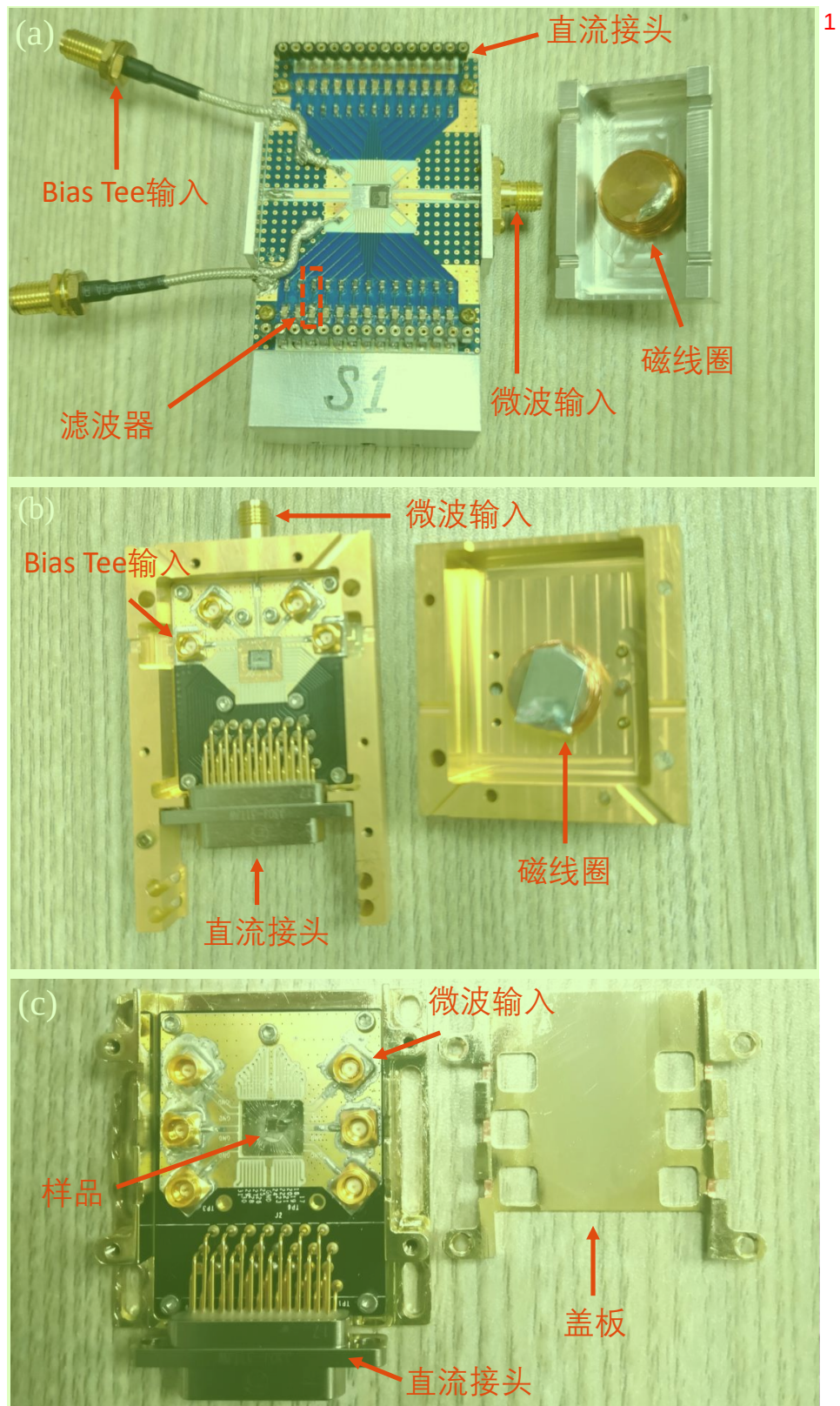
图 3.5 不同版本的样品盒，自上而下分别为第一代、第二代和第三代。 2
