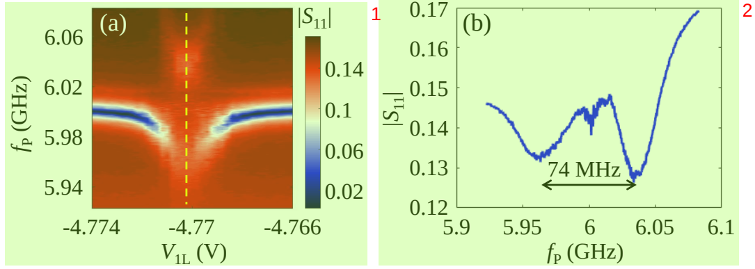
图 3.13 (a) DQD1 的量子点间隧穿速率 2t_c/\hbar 接近腔频 \omega_r 时的真空 Rabi 劈裂。(b) 在失谐量为 0 处扫描的频谱，可以提取得到耦合强度 2g_0/2\pi = 74 MHz。
