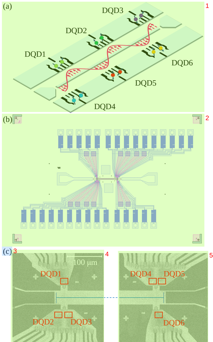
图 7.1 谐振腔耦合的半导体量子点六比特。(a) 耦合结构示意图。(b) 耦合结构设计图。(c) 六比特样品的扫描电子显微镜图。
