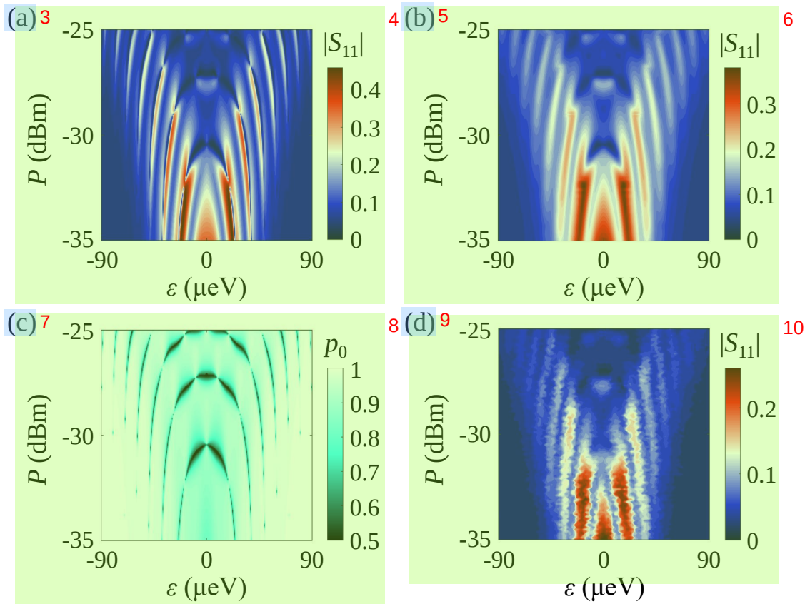
图 6.7 (a) 驱动频率 f_d = 2.27 GHz 在接近三分之一谐振频率处的理论预言结果，驱动功率 11 P = -29 dBm，对应幅值 A_d = 45 \mu\text{eV} 。(b) 相同的数值计算，但是额外考虑了失谐量 \varepsilon 具有 2.5 \mu\text{eV} 的噪声展宽。(c) 理论计算的 Floquet 态 |\phi_0\rangle 平均布居。(d) 驱动频率 f_d = 2.27 GHz 时的谐振腔响应实验结果。
